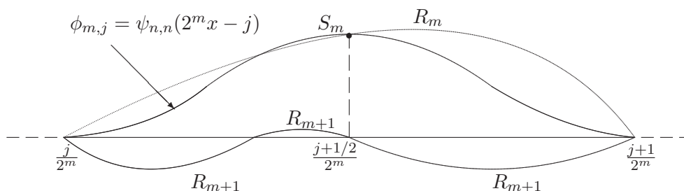
Рис. 2. Процесс приближения по остаткам Fig. 2. Approximation process by residual
