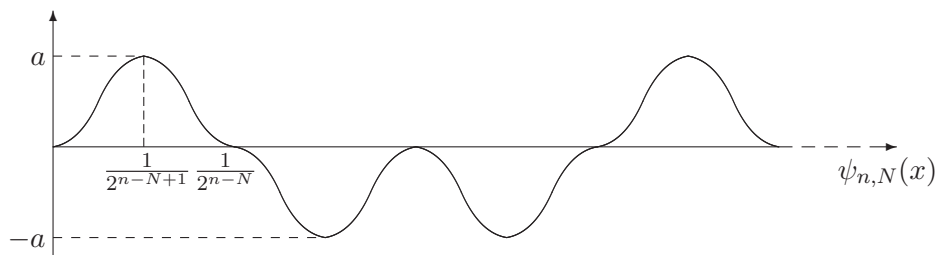
Рис. 1. Двоичный базисный сплайн / Fig. 1. Binary basic spline
